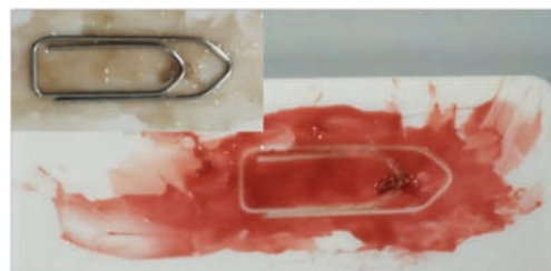
Şekil 2. Işıkla renk değiştiren (fotokromik) farklı maddelerin sahip oldukları renkler: UV ışığına maruz kalmadan önce (küçük resim) ve sonra (büyük resim).
